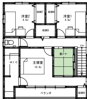
2階平面図
