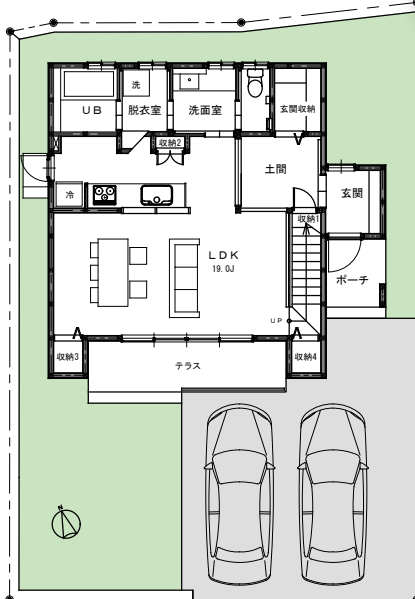
1階平面図
